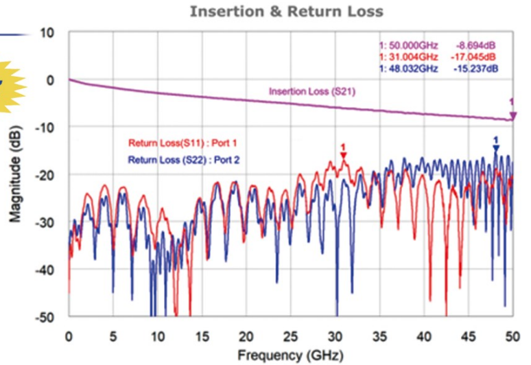
S-parameter
